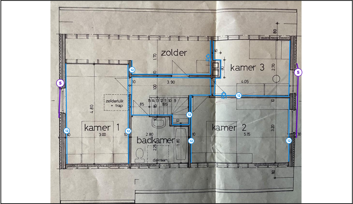
Legende van plan 1.5: Verdiep - muren
